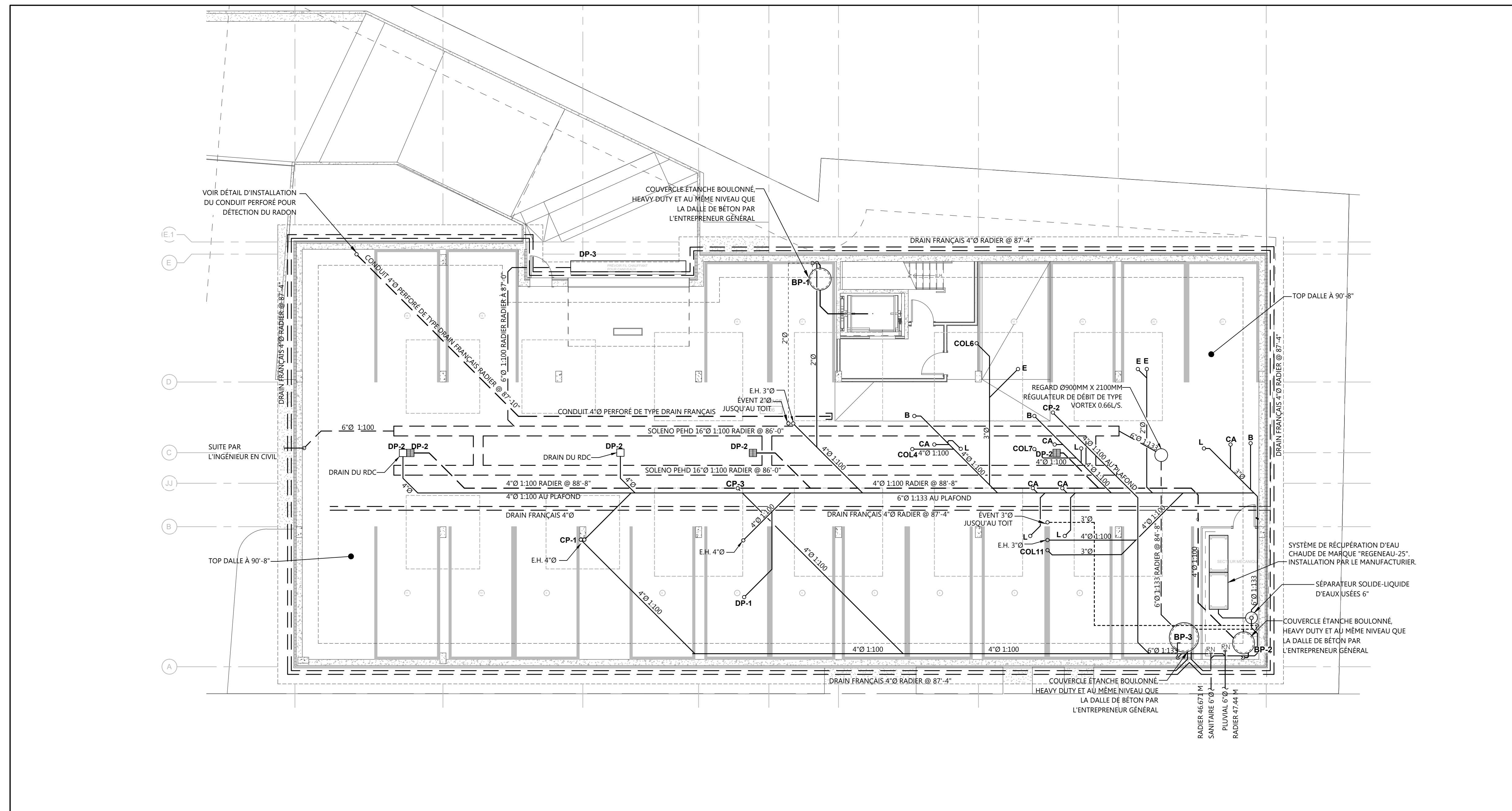
DRAINAGE : SOUS-SOL ÉCHELLE : 1/8" = 1'-0"
