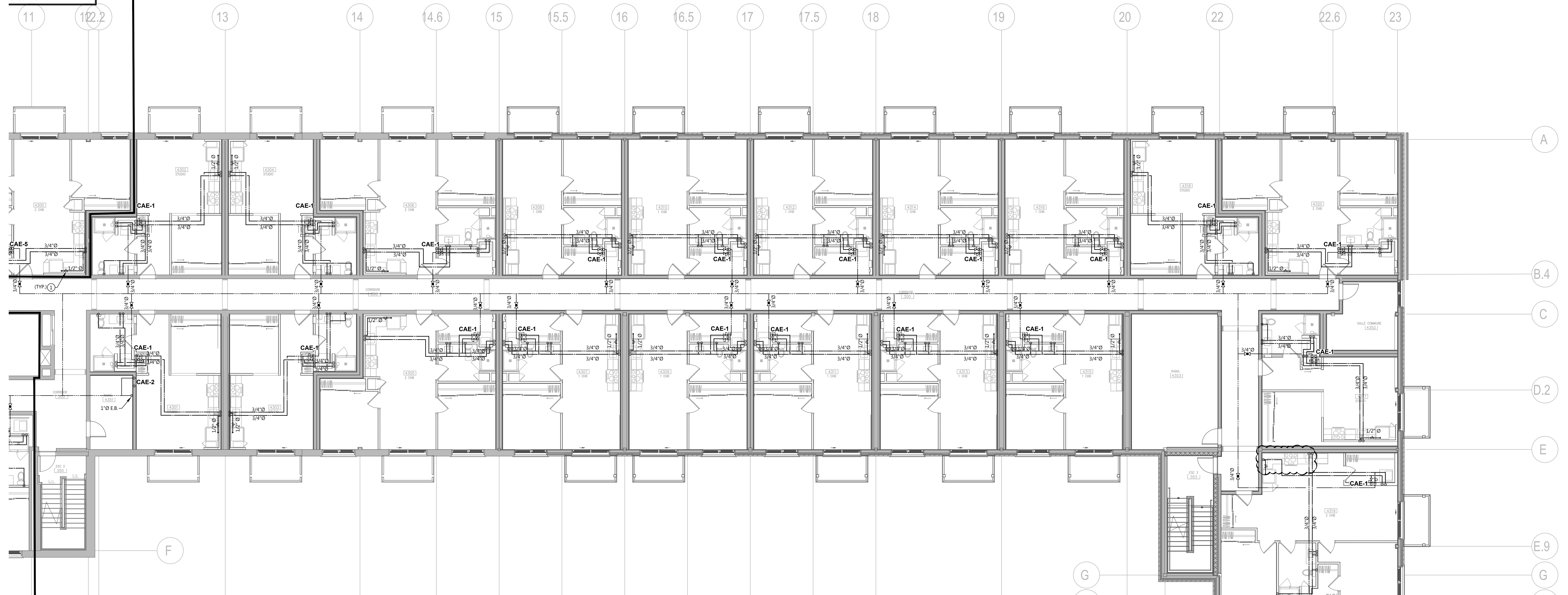
PLAN D'AMÉNAGEMENT EAU DOMESTIQUE : NIVEAU 3 PARTIE DROITE ÉCHELLE: 1/8"=1'-0"
